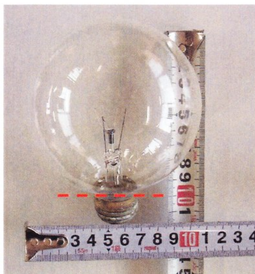
落下したものと同種の電球 ※赤点線位置でソケット部分から外れて落下
