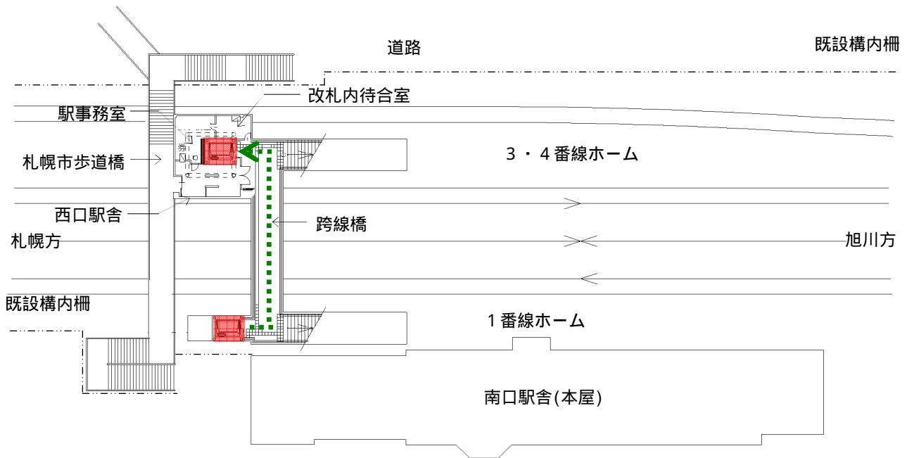
西口駅舎及び跨線橋階(2階)平面図
