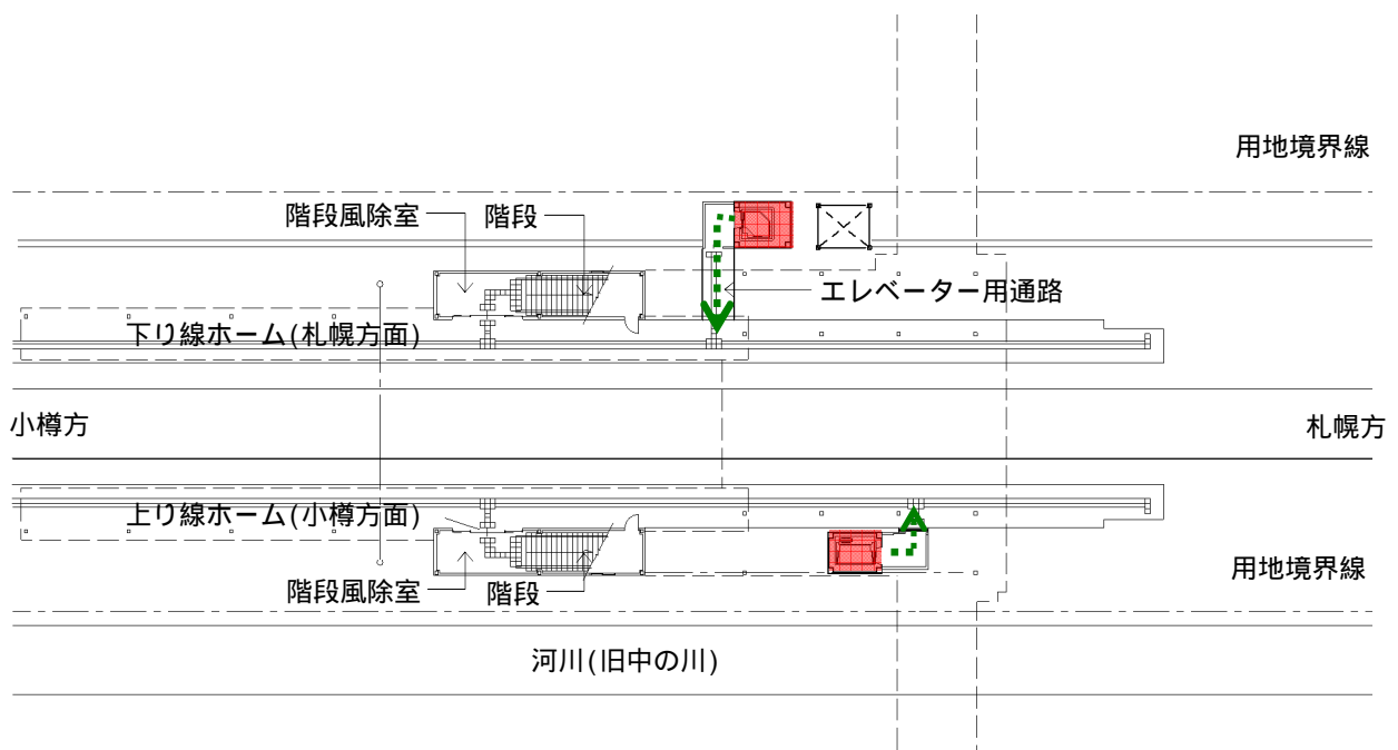
ホーム階(1階)平面図
