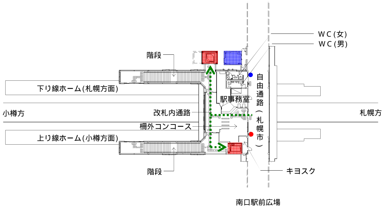
駅舎階(2階)平面図
