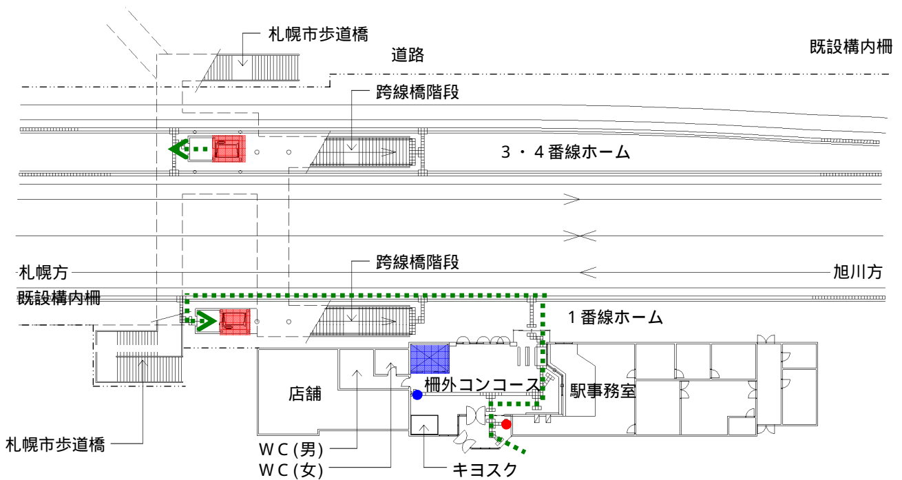
南口駅舎階(1階)平面図
