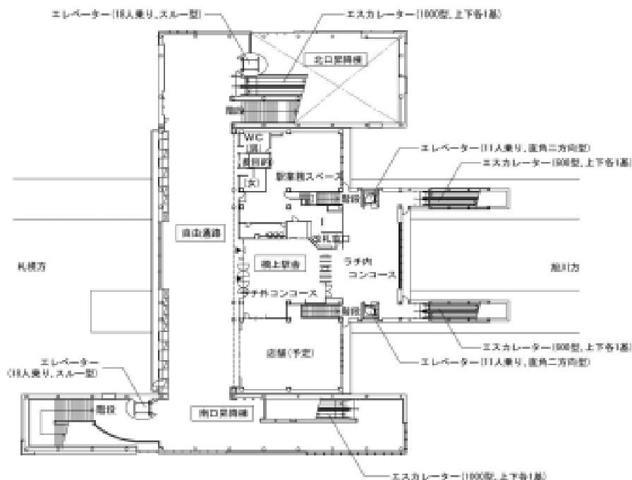
2階平面図
