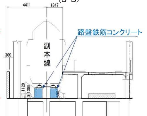
断面图 (B-B)
