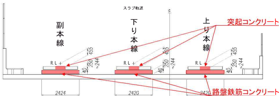
断面图 (A-A)
