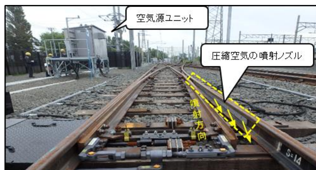
圧縮空気式除雪装置の設置例
