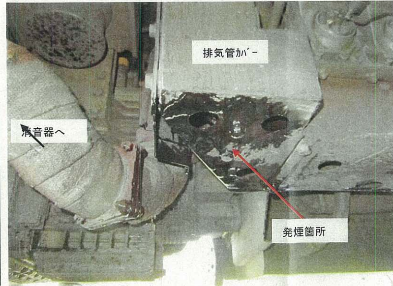
排気管カバー 下部
