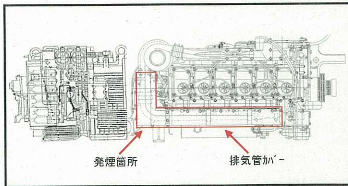
No. 2機関 正面図
