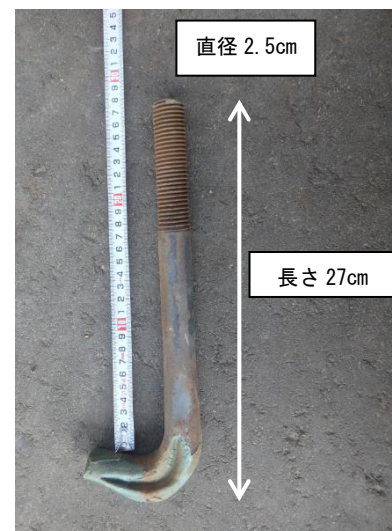
写真2 落下したフックボルト
