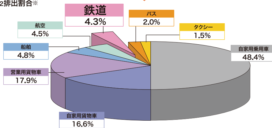
運輸部門のCO 2 排出割合※
