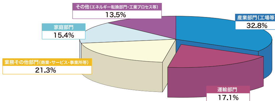
日本における部門別のCO 2 排出割合※
